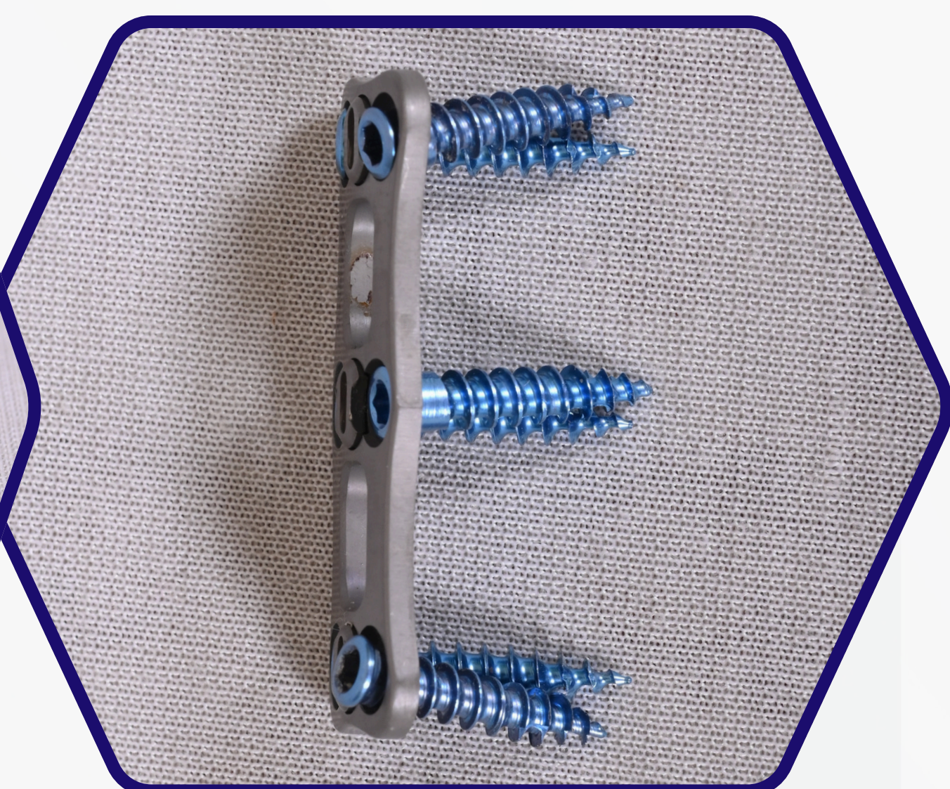
ANTERIOR CERVICAL PLATING SYSTEM
